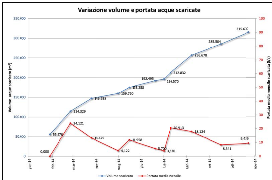
Grafico 11: portate emunte dal laghetto di cava
