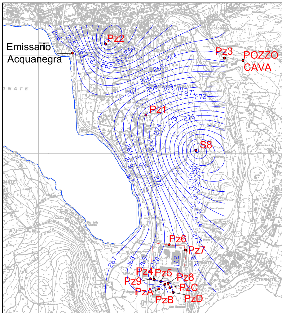
Figura 1: andamento piezometrico 23 ottobre 2014
