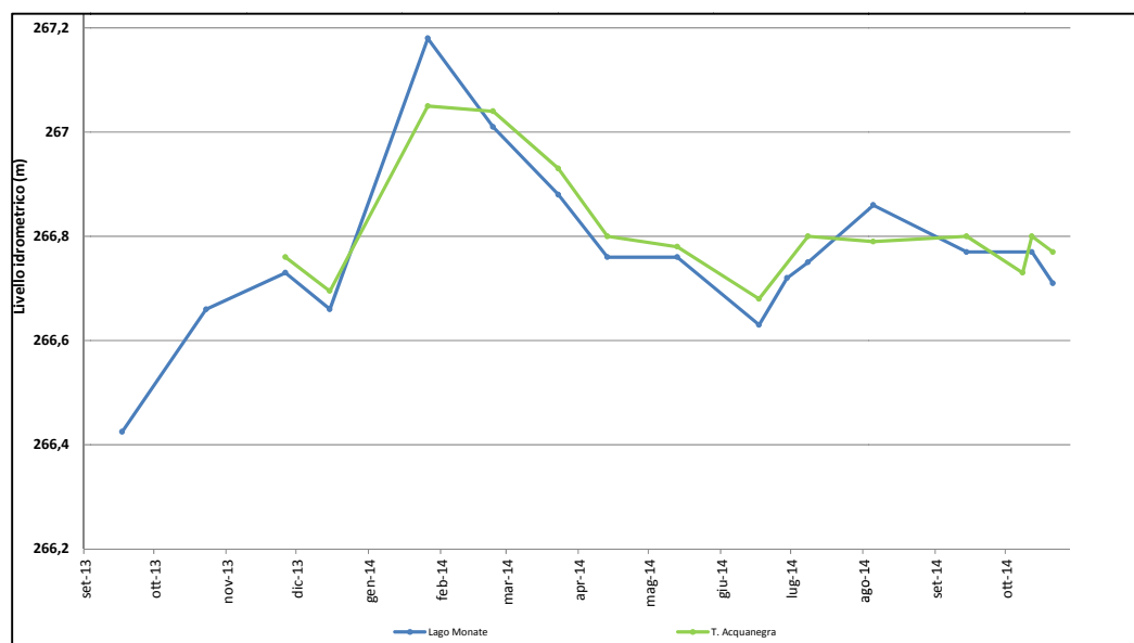
Grafico 8: confronto livelli idrometrici Lago Monate-Torrente Acquanegra
