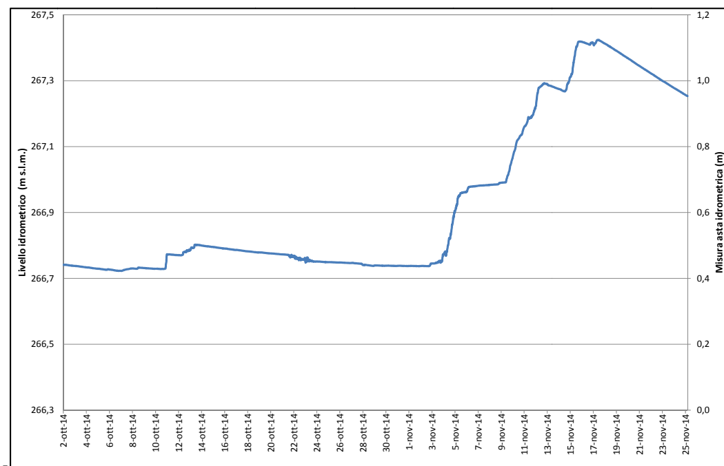
Grafico 7: oscillazione livello idrometrico Torrente Acquanegra
