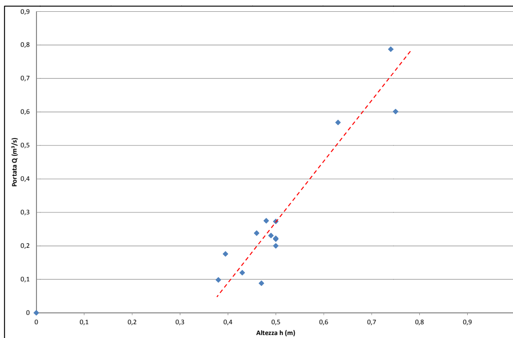
Grafico 10: scala deflusso - portata
