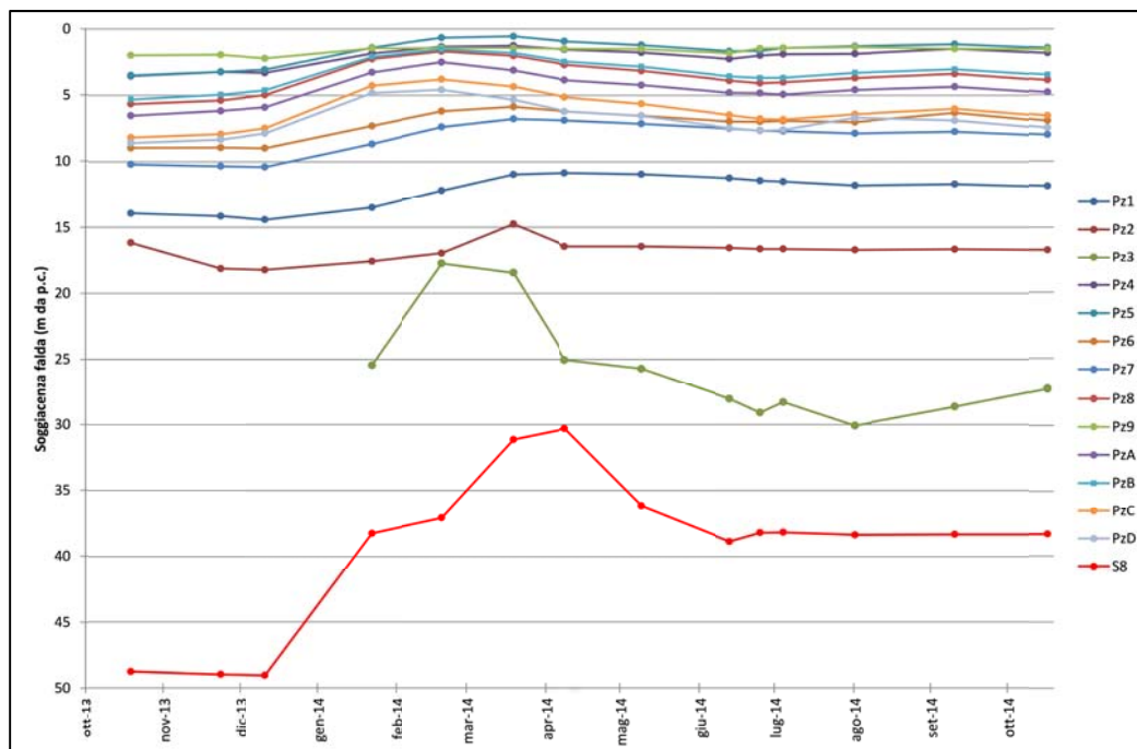
Grafico 6: oscillazione piezometriche (ottobre 2013 – ottobre 2014)
